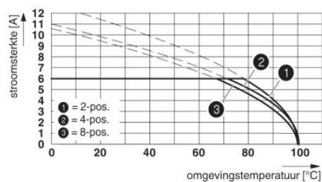
Deratingcurve voor: PTSM 0,5/...-P-2,5 met PTSM 0,5/...-HH-2,5-THR R..
