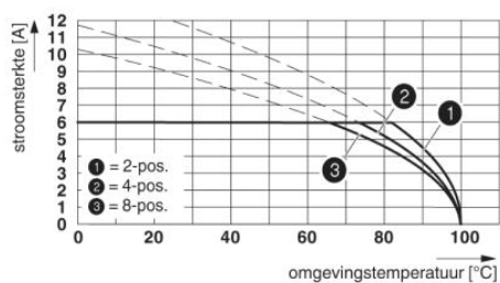
Deratingcurve voor: PTSM 0,5/...-P-2,5 met PTSM 0,5/...-HV-2,5-THR R...
