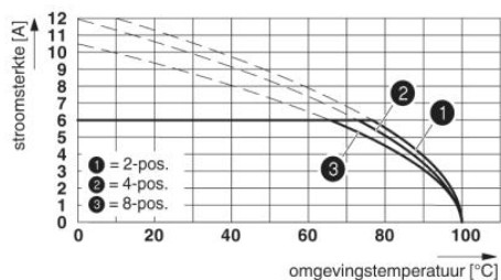
Deratingcurve voor: PTSM 0,5/...-P-2,5 met PTSM 0,5/...-HV-2,5-THR R...
