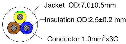
A-A
